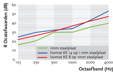
Isomat KE gelijmd op 1 mm staalplaat
