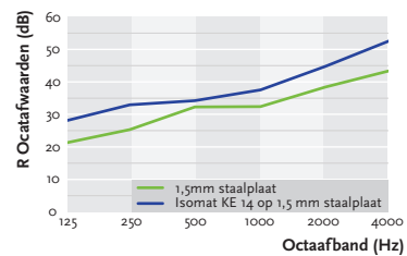
Isomat KE gelijmd op 1,5 mm staalplaat
