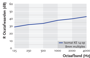
Isomat KE gelijmd op 8 mm multiplex
