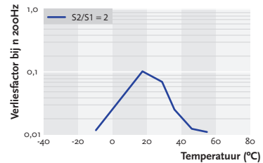
Verliesfactor van Vibradamp A90-P van de temperatuur, 2x dikte van staalplaat aangebracht
