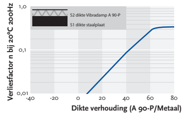
Verliesfactor van Vibradamp A90-P als functie van de verhouding laagdikte/plaatdikte
