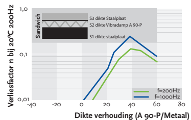
Verliesfactor van Vibradamp A90-P als functie van de temperatuur, 'sandwich' toegepast in de verhouding S1:S2:S3 = 4:1:1
