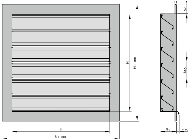
Tekening met maatvoeringen van standaard WG-rooster
